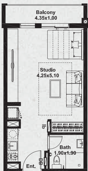
ST/B
